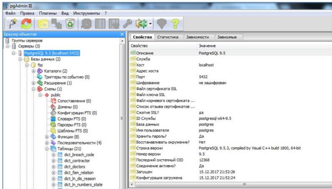
Рисунок 31 – Сервер PostgreSQL 9.5
