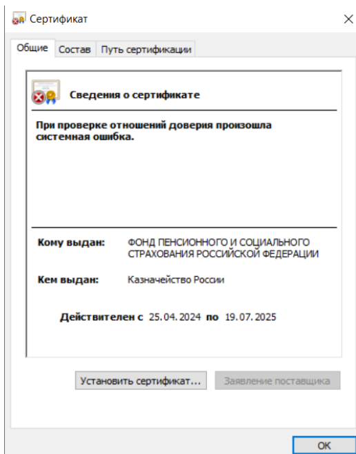
Рисунок 13 – Установка сертификата
