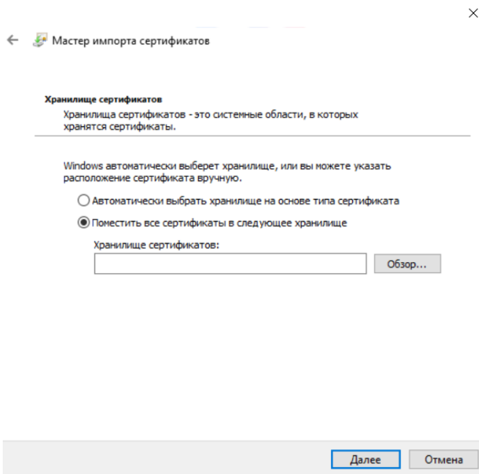
Рисунок 15 – Хранилище сертификатов
